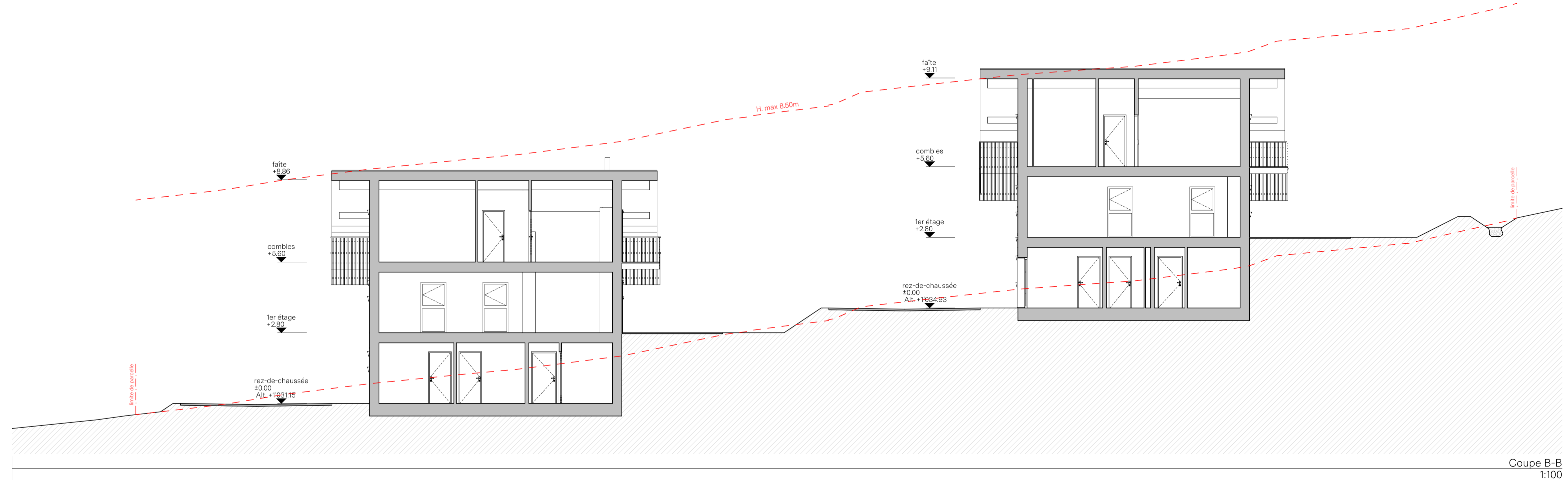
Coupe A-A 1:100
