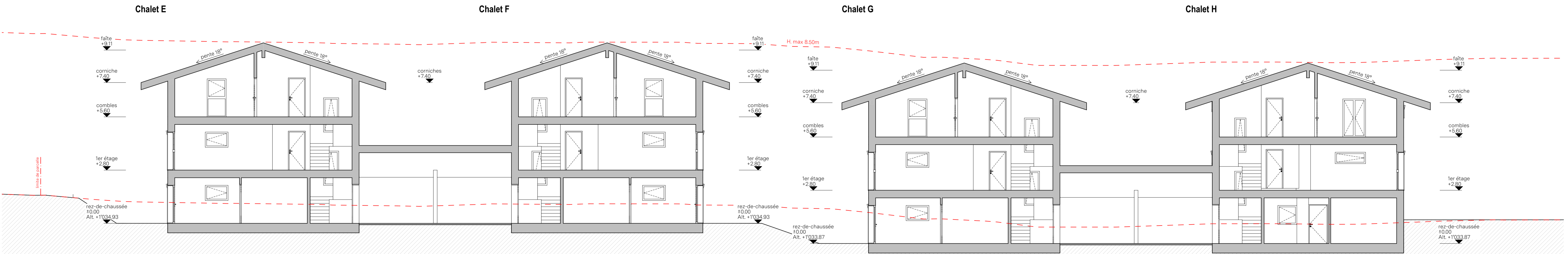
Coupe E-E 1:100
